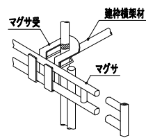
マグサ取付詳細図
